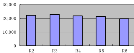
発電量 (MWh)
